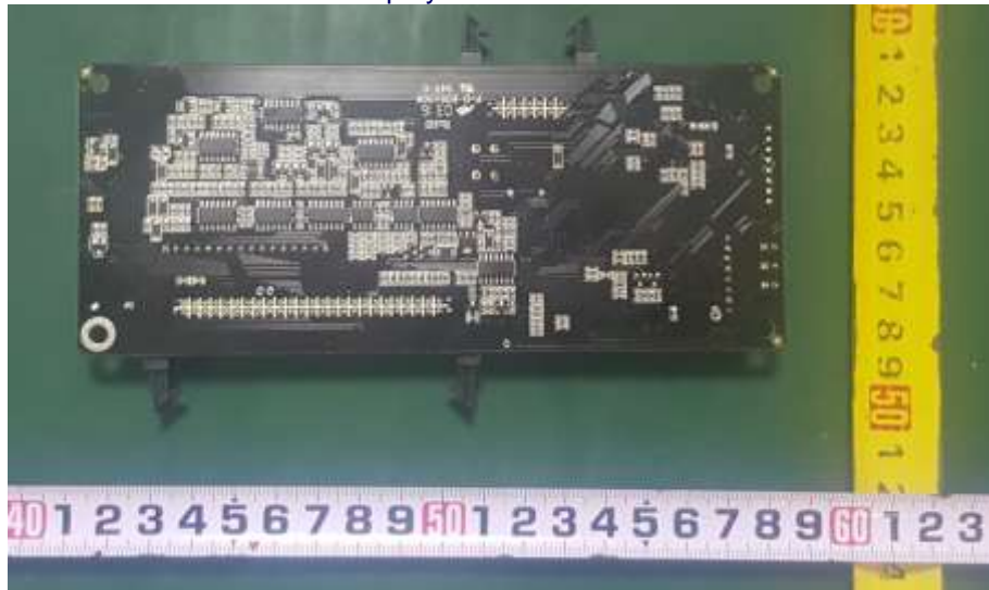
BLD-3K-TL3, BLD-3.5K-TL3, BLD-4K-TL3, BLD-5K-TL3 - Display board-Solder side
